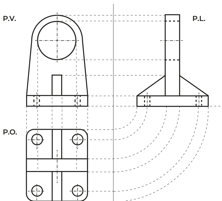
Proiezione ortogonale dell'oggetto
