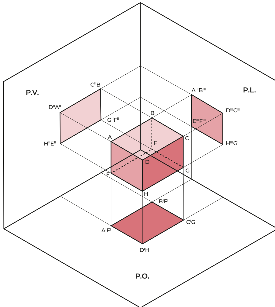
Schema di riferimento per la proiezione di un oggetto su tre piani
